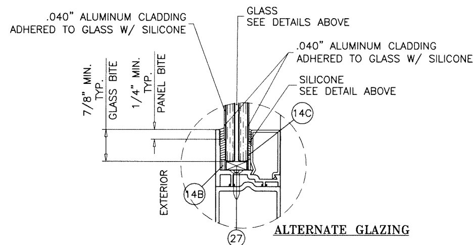
GLAZING OPTIONS
