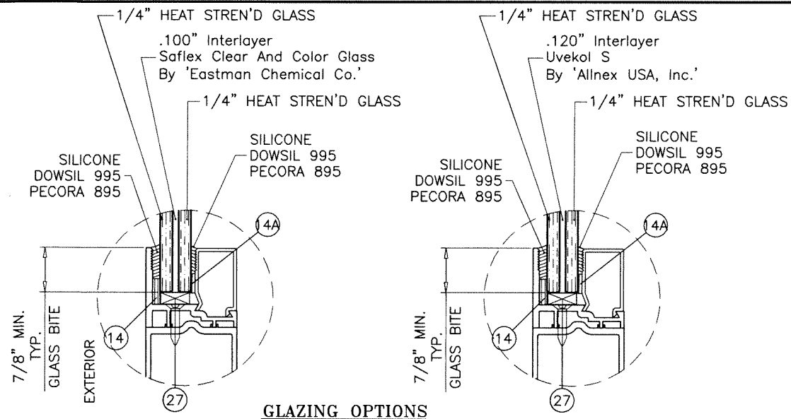
GLAZING OPTIONS
